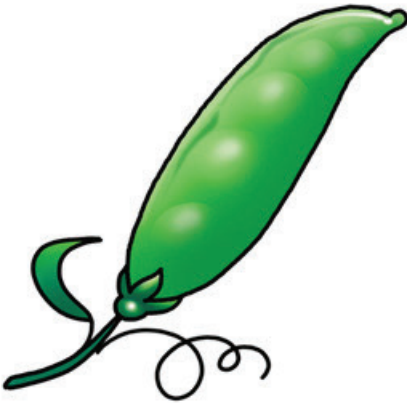
Peas
